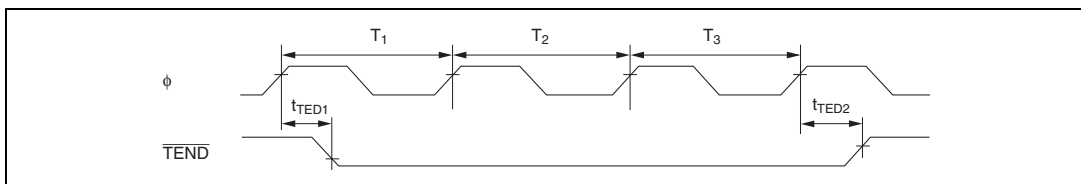
図 21.25 DMAC \overline{\text{TEND}} 出力タイミング / 3 ステートアクセス
