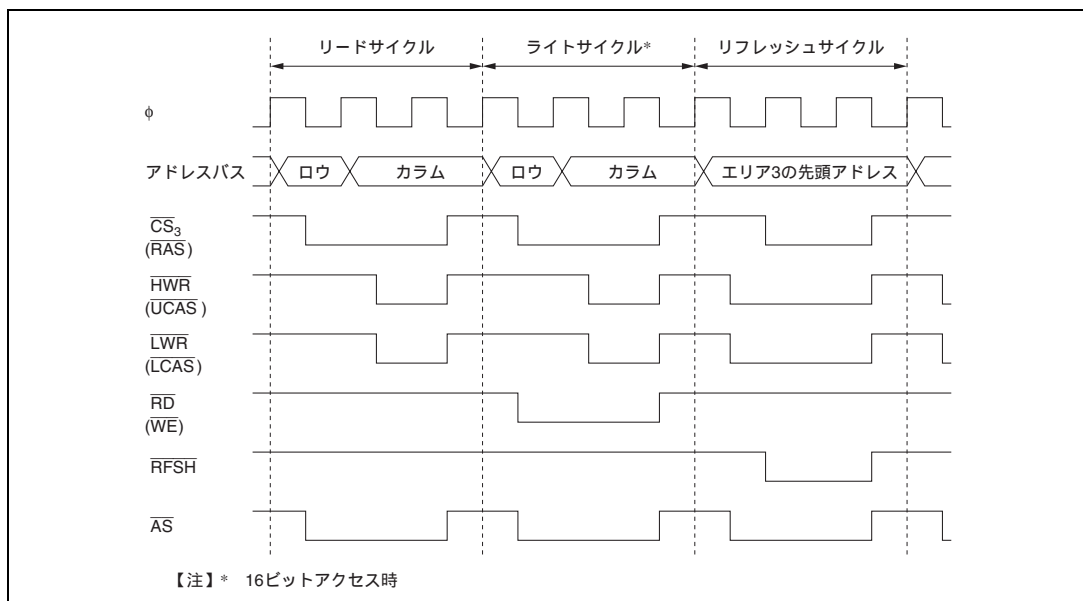
図 7.5 DRAM 制御信号出力タイミング (2) ( 2\overline{\text{CAS}} 方式)
