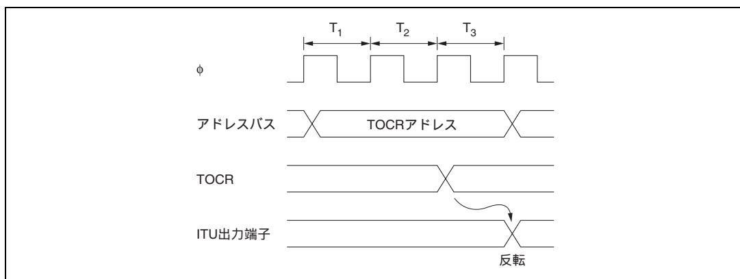
図 10.56 TOCR へのライトによる ITU 出力レベル反転タイミングの例
