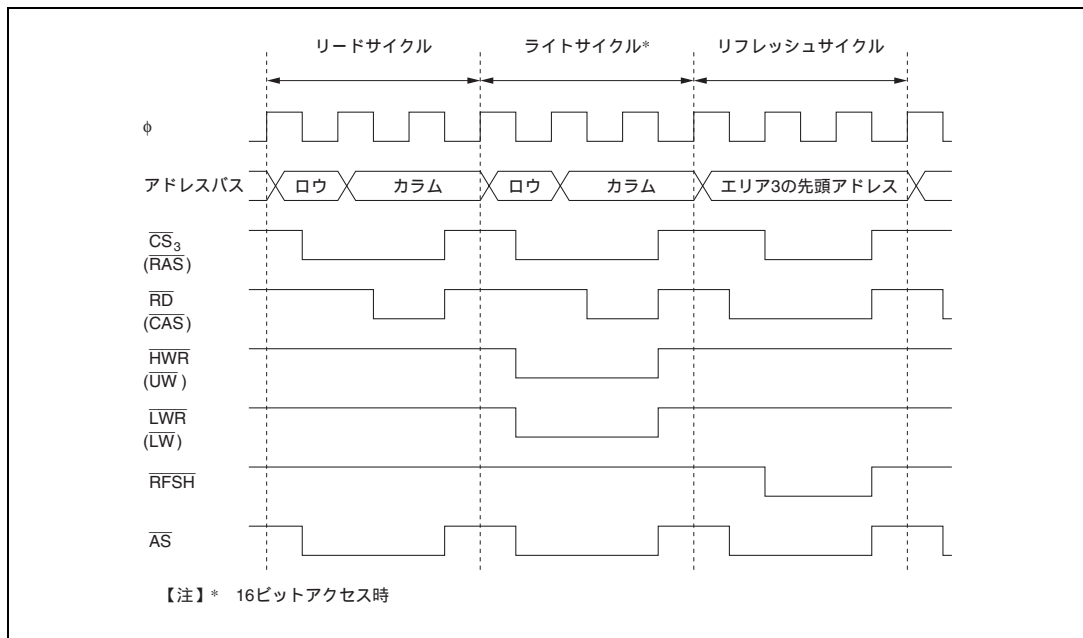
図 7.5 DRAM 制御信号出力タイミング (1) ( 2\overline{\text{WE}} 方式)
