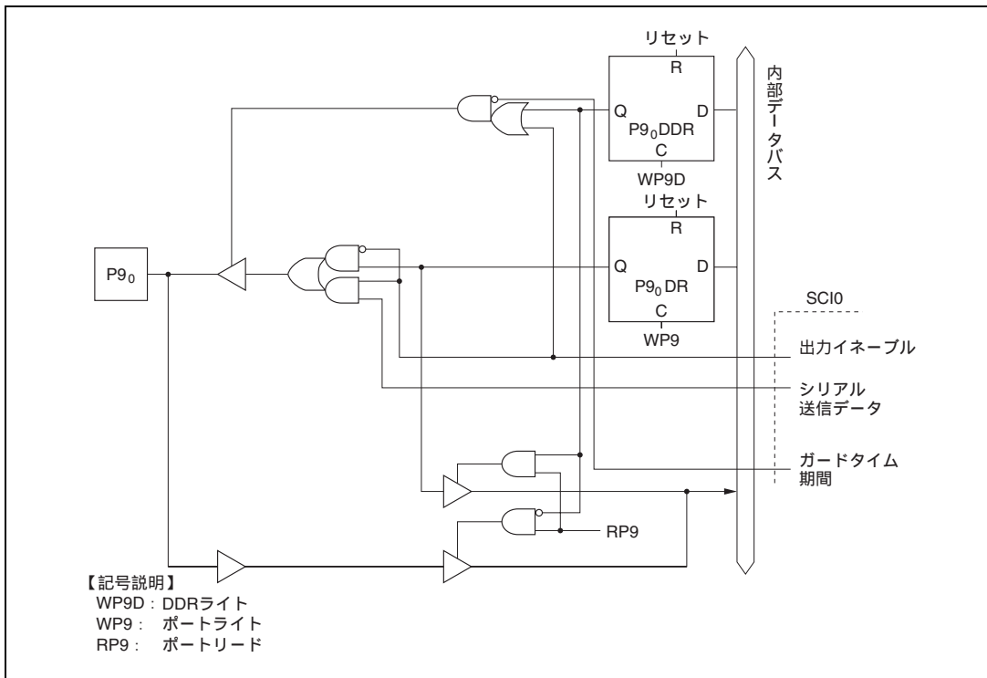
図 C.9 (a) ポート9ブロック図 (P9 0 端子)
