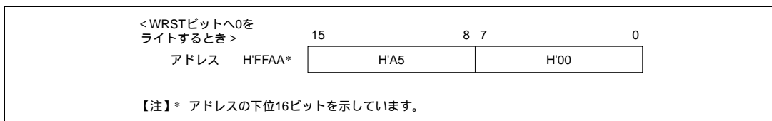
図 12.3 RSTCSR へのライトデータ
